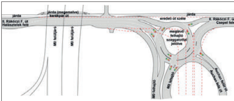
A tervezett M0 halásztelki lehajtó és felhajtó a Csepel felé eső oldalon.
